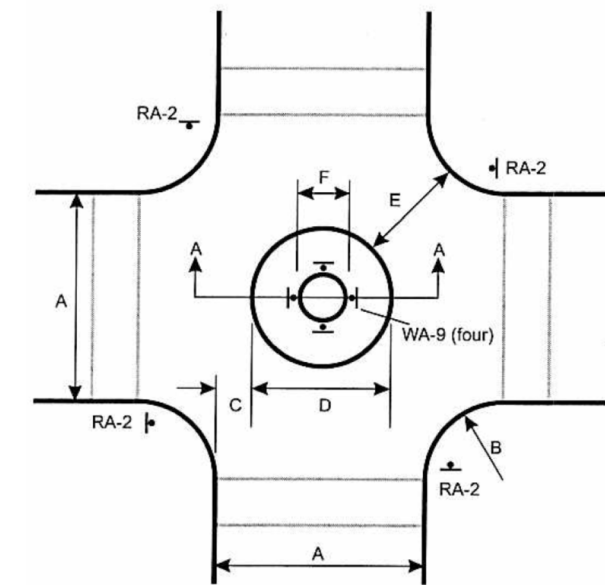
Figure 2.6 (7) Mini Traffic Circle
